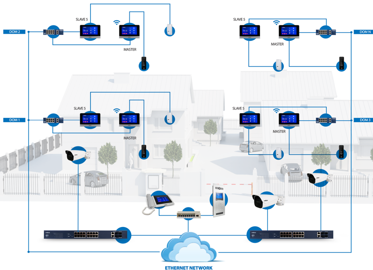
NVE-M200WIFI NVE-M200LITE Monitor abonencki
