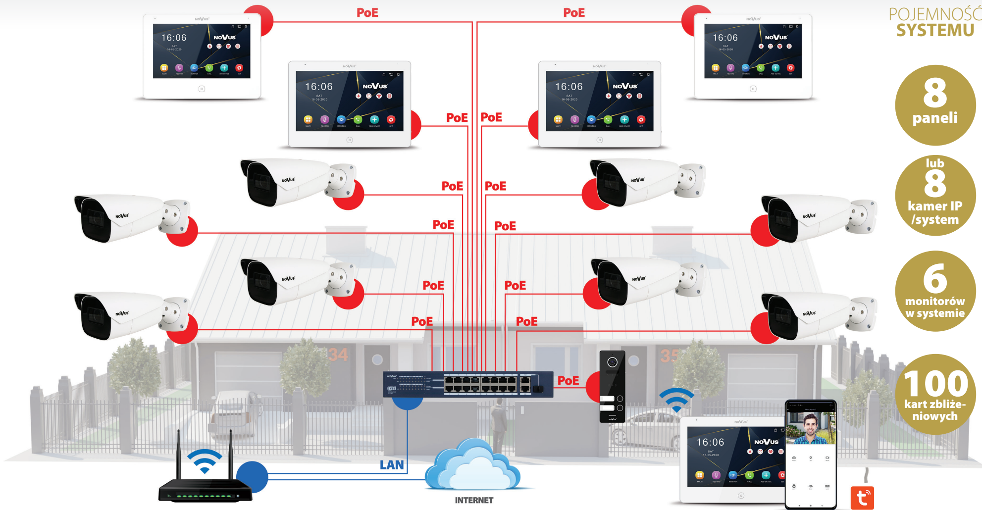
NVE-EPV102P Panel wejściowy IP
